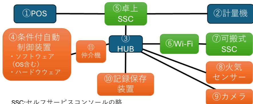
図1 条件付自動制御システムの構成機器
