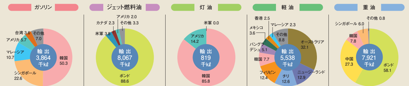
■主要石油製品の国別輸出比率(2023年度)
